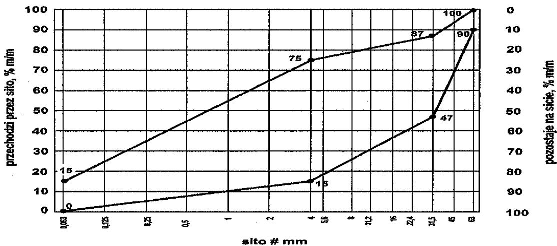
Rysunek 2. Mieszanka kruszyw 0/63 do górnej warstwy podłoża ulepszego
